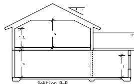
Sektion B-B (Sektion B-B visar med inreklädd burspråk)
